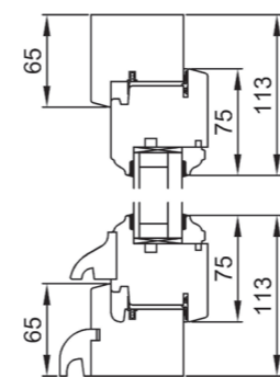
Coupe verticale
